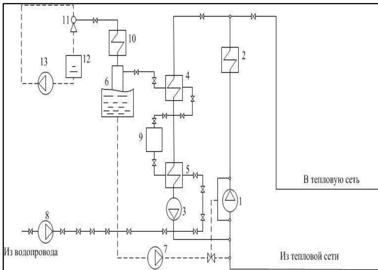
Рисунок 1.2.6.1 – Принципиальная тепловая схема котельной с водогрейными котлами
