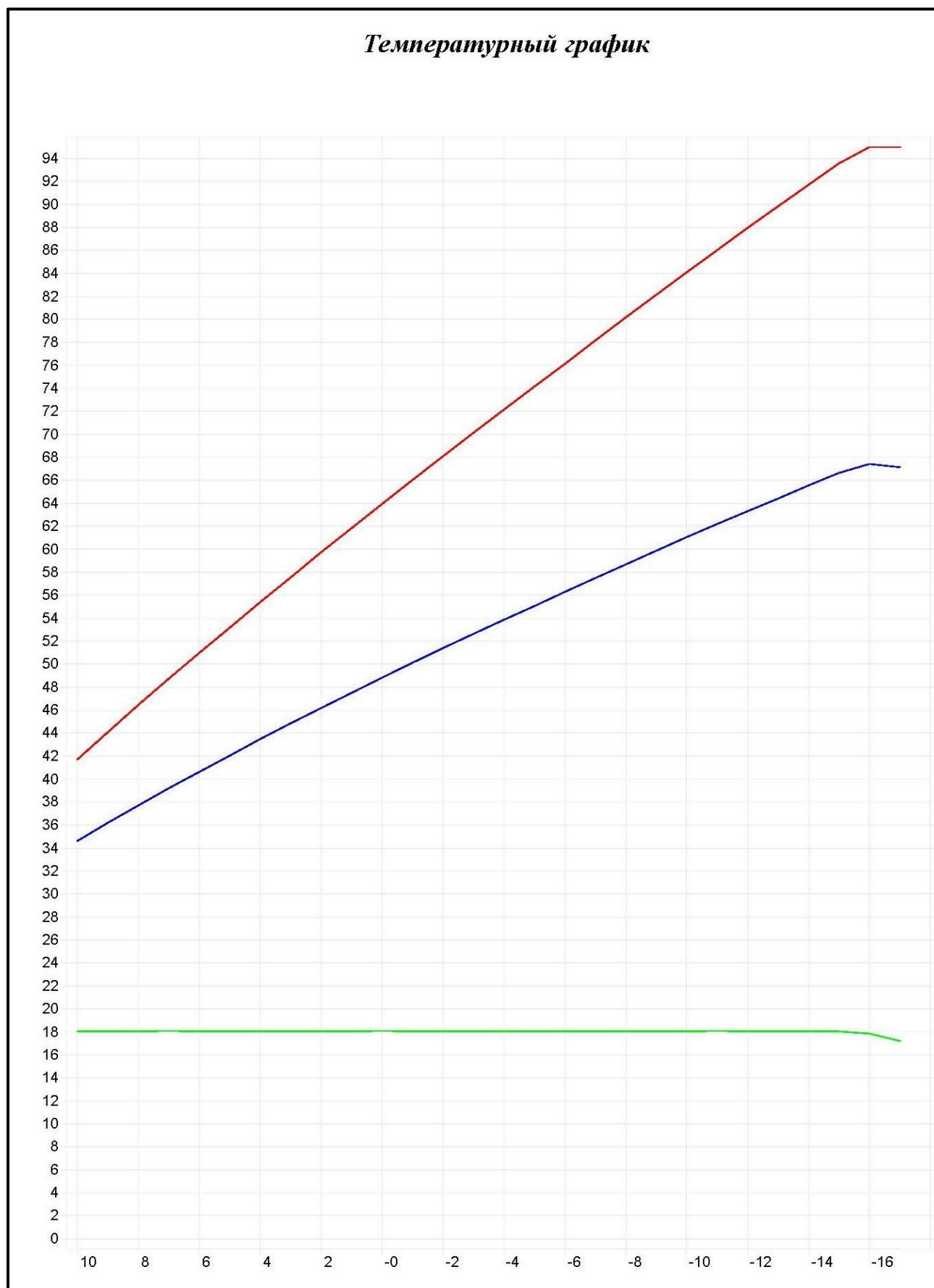
Рисунок 1.2.7.1 – График изменения температур теплоносителя 95–70 °С
