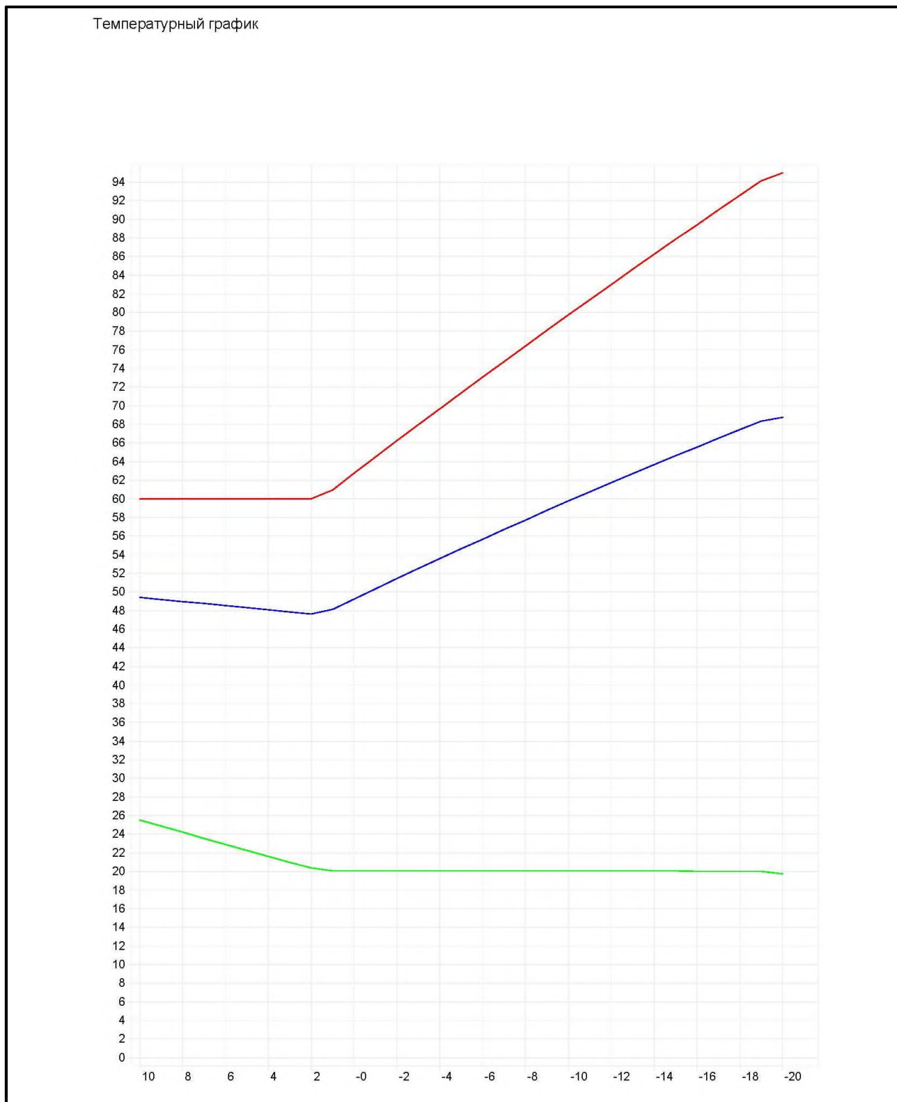
Рисунок 1.2.7.1 – График изменения температур теплоносителя 95–70 °С
