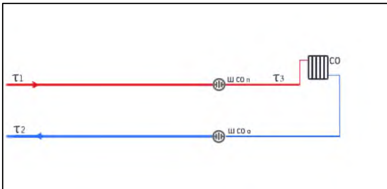
Рисунок 1.3.16.1 – Схема присоединения потребителей «Потребитель с непосредственным присоединением СО»
