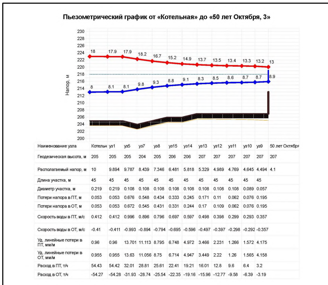
Рисунок 1.3.8.1 – Пьезометрический график по пути: Котельная с. Октябрьское – ул. 50 Лет Октября, б/н
