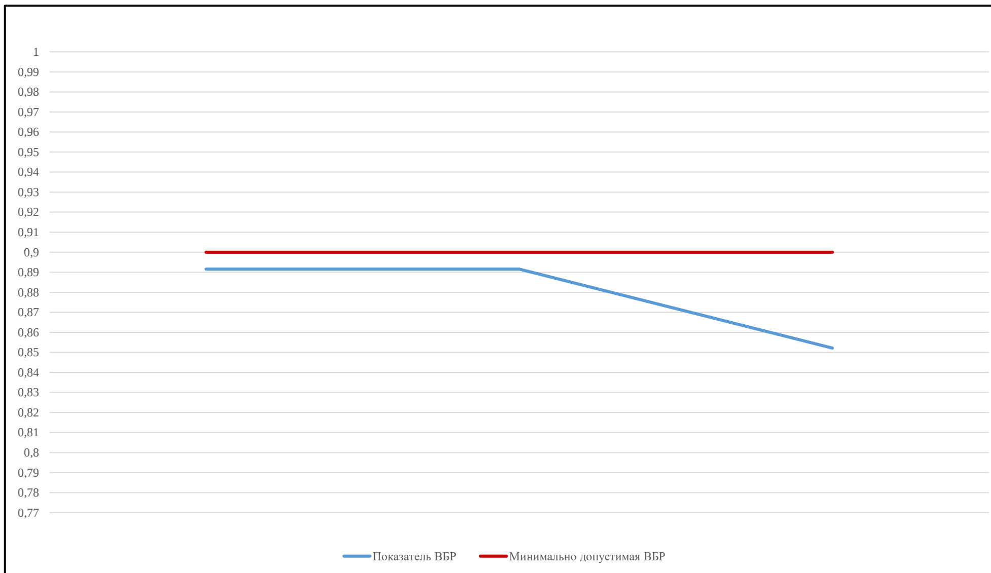
Рисунок 11.3.1 – ВБР сетей Котельной с. Октябрьское
