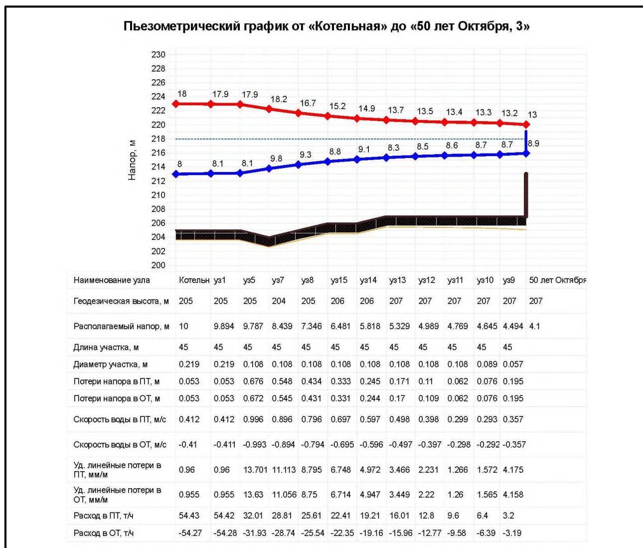
Рисунок 4.2.1 – Пьезометрический график Результаты гидравлического расчёта приведены в приложении 1.
