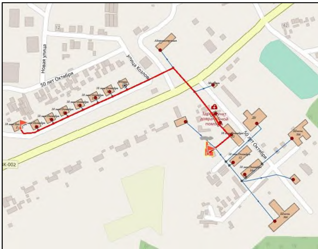
Рисунок 1.3.8.2 – Путь для пьезографика: Котельная с. Октябрьское – ул. 50 Лет Октября, б/н
