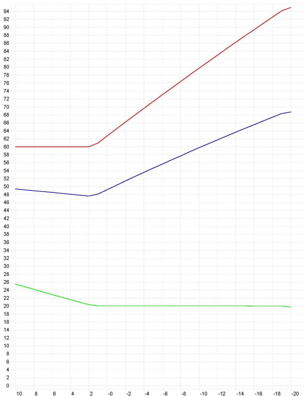
Рисунок 5.8.1 – Расчет отпуска тепловой энергии для котельной с. Октябрьское в течение года при температурном графике 95-70 °С
