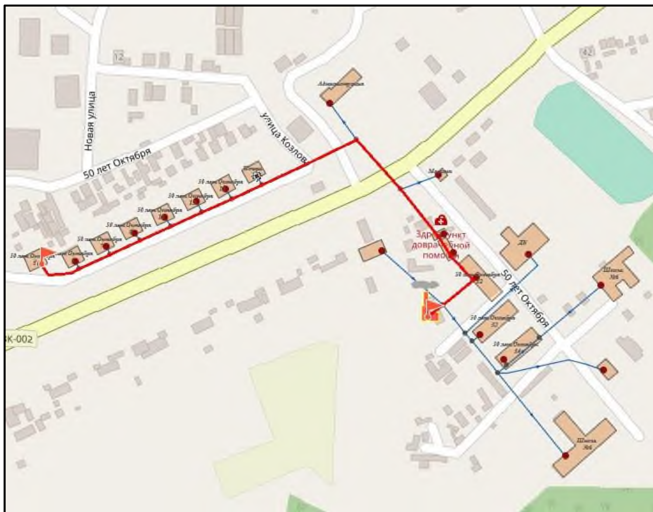
Рисунок 1.3.8.2 – Путь для пьезографика: Котельная с. Октябрьское – ул. 50 Лет Октября, д. 3
