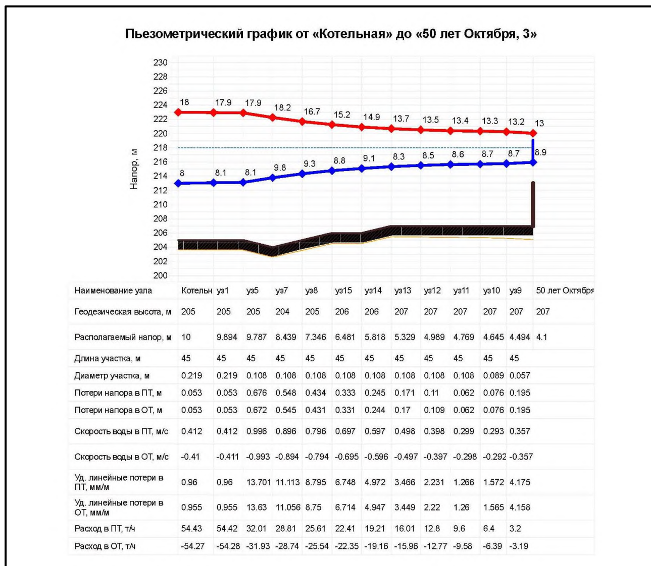
Рисунок 1.3.8.1 – Пьезометрический график по пути: Котельная с. Октябрьское – ул. 50 Лет Октября, д. 3
