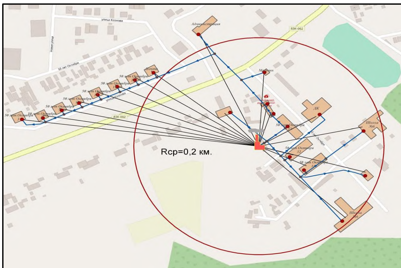
Рисунок 2.5.1 – РЭТС Котельной с. Октябрьское
